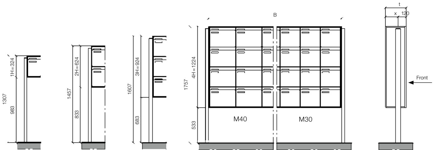
Stützen- montage eckig
