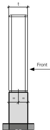
Sockelmontage
