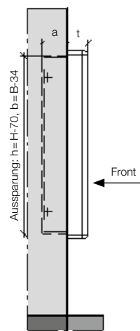
Teilweiser Mauereinbau
