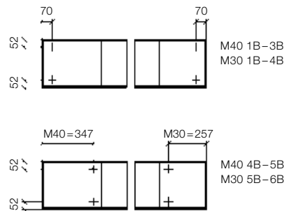
Befestigungspunkte Wandanbau Verkleidung eckig
