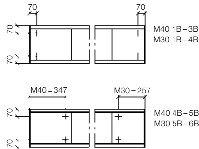
Befestigungspunkte Wandanbau Verkleidung rund/schräg
