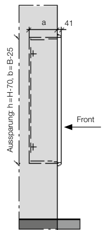
Mauereinbau
